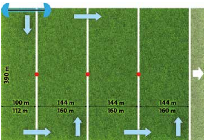
Monostar mit beidseitigem Überhang, ermöglicht Streifenbreiten bis zu 160m.
